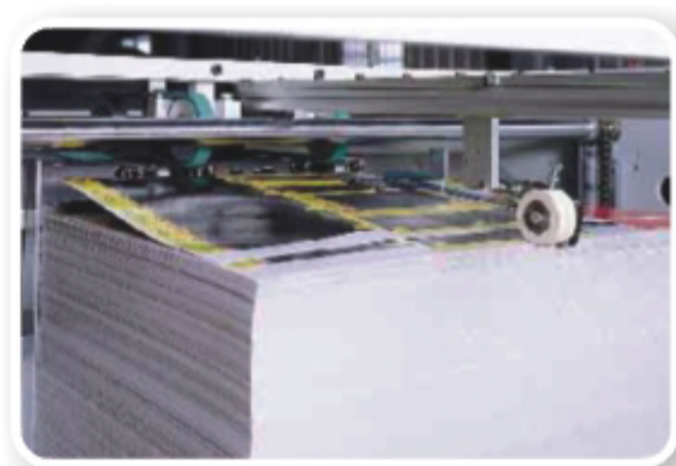
LITHO SHEET FEEDER 前緣送紙式面紙飛達
