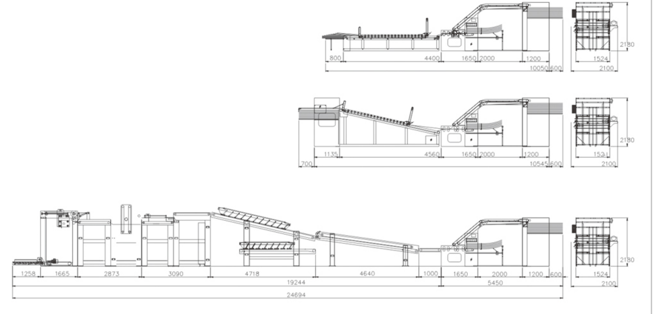
MACHINE LAYOUT 設備示意圖： * LAYOUT SHOWS ASPIRE CS-1416 設備尺寸展示型號 ASPIRE CS-1416
